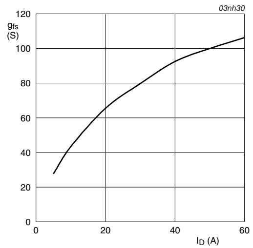
T_j = 25^\circ C; V_{DS} = 25V
