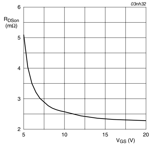
T_j = 25^\circ C; I_D = 25A
